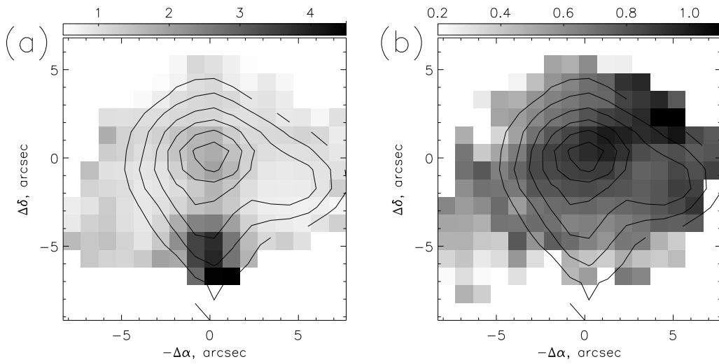
Рис. 3.11 Карта отношений линий [\text{OIII}]\lambda 5007/\text{H}\beta (слева) и [\text{SII}]\lambda 6731/6717\text{\AA} (справа) в Mrk 334. Наложены изофоты в линии [\text{OIII}]\lambda 5007 . Для линий серы более темные цвета соответствуют более высокой электронной плотности.
