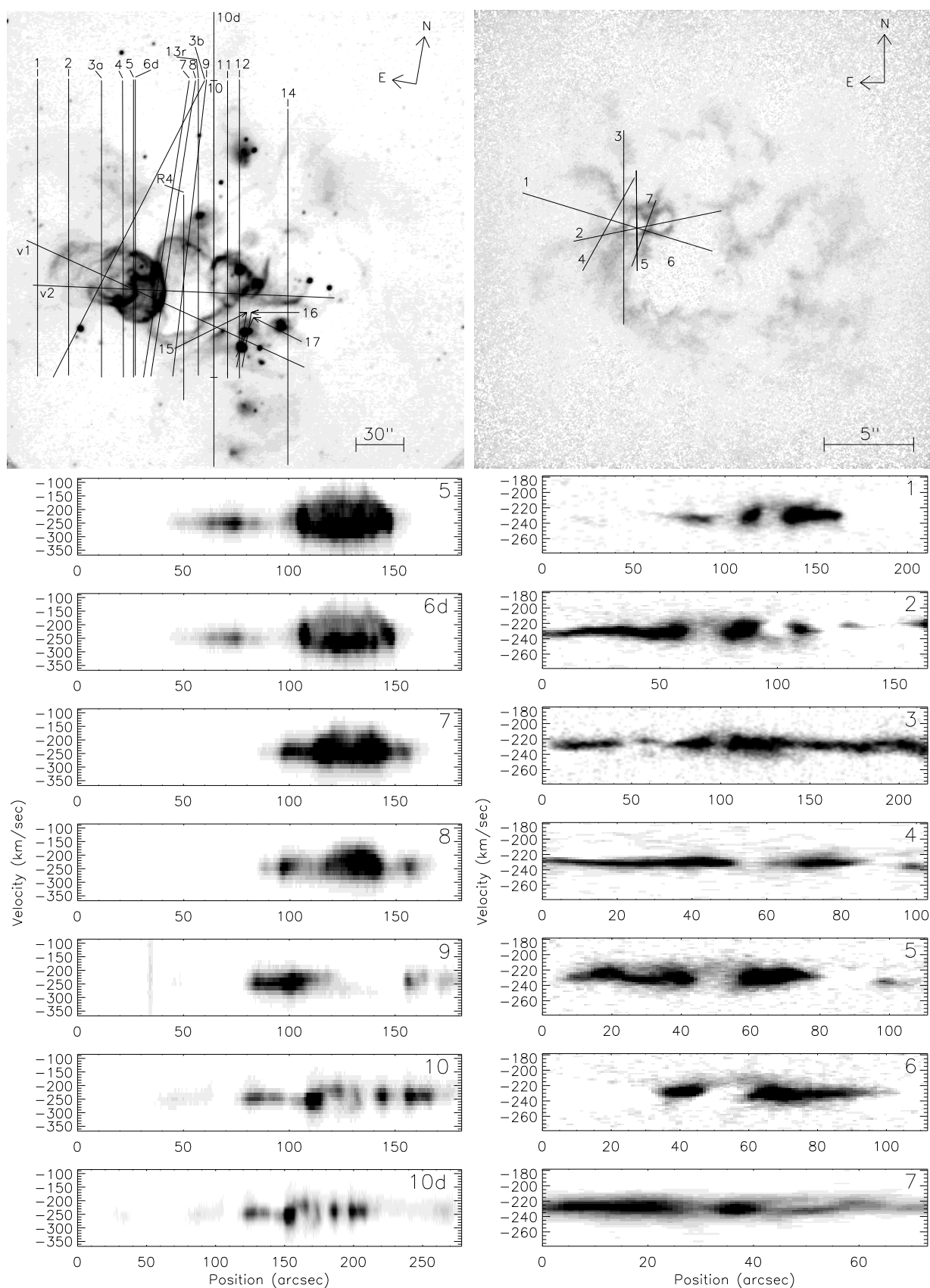
Рис. 6.3 Примеры PV-диаграмм в оболочечном комплексе IC 1613 (Лозинская и др., 2003). Слева – ионизованный газ ( H\alpha , ИФП), справа – HI (VLA). Вверху показано расположение разрезов, вдоль которых строились диаграммы, нанесенных поверх соответствующих распределений яркости.
