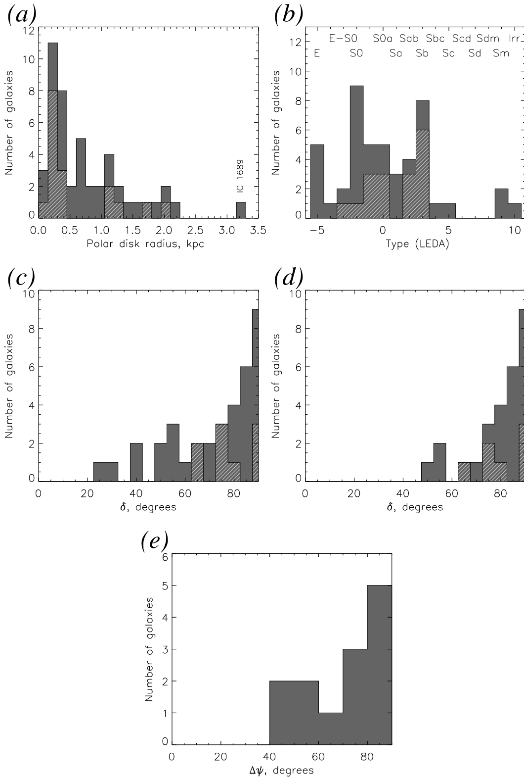
Рис. 5.8 Гистограммы распределения внутренних полярных структур по размерам (а) и морфологическим типам галактики (b). Серым цветом показаны все галактики, штриховкой – только с барами и трехосными балджами. Ниже показаны распределения по углу наклона ВПС к основному диску галактики: (c) – весь возможный диапазон решений для \delta из (2.1), (d) – в случае двух решений – бралось большее. (e) – распределение по углу между большой осью полярного диска и бара (трехосного балджа).
