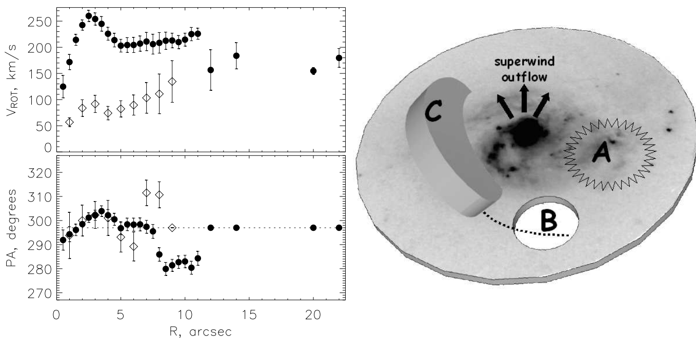
Рис. 3.13 Слева – кривая вращения Mrk 334 и вариации PA_{kin} с радиусом. Черные кружки – измерения по полю скоростей, полученным с ИФП в H \alpha , ромбы – измерения по полю скоростей звездного компонента. Справа – схема, поясняющая пространственную структуру внутренней ( r < 5 кпк) области Mrk 334, пунктиром отмечена предполагаемая орбита ядра спутника.
