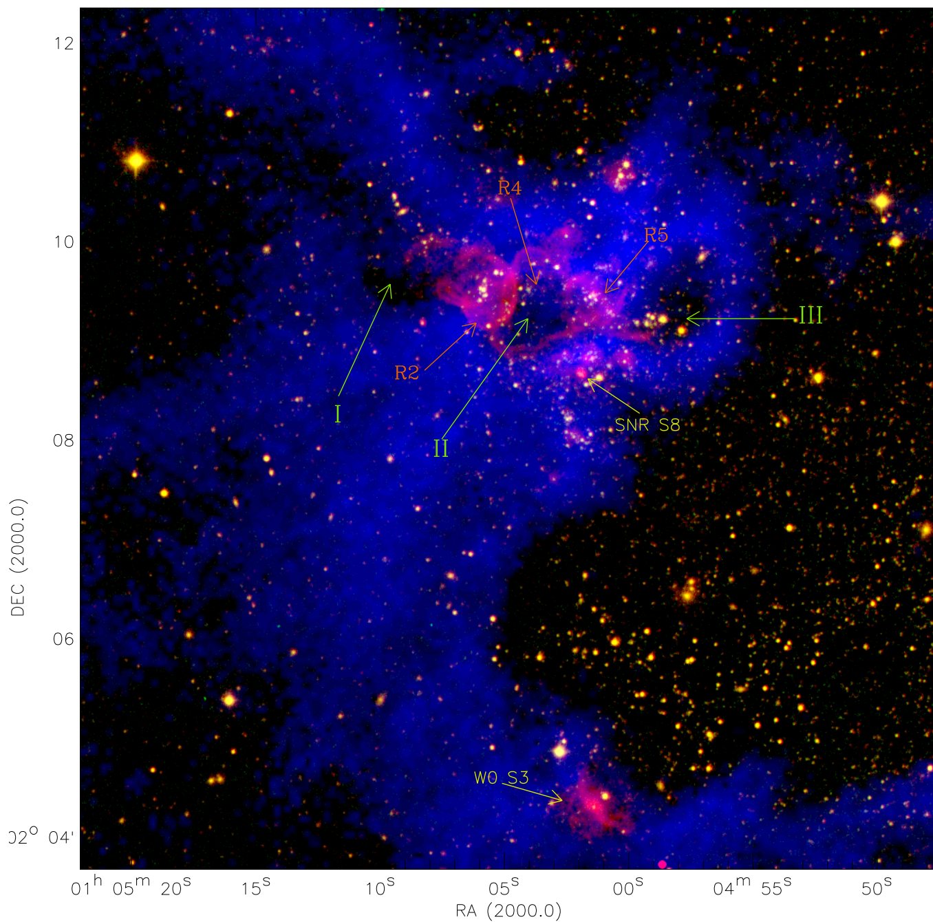
Рис. 6.2 Композитное изображение восточной половины IC 1613. Синим показано распределение HI (VLA), красным и золотистым – изображение в эмиссионной линии H\alpha и в континууме (1-м телескоп “Цейсс-1000” САО РАН с редуктором SCORPIO). Стрелочками отмечены упомянутые в тексте объекты. Желтым – туманность вокруг звезды WO и остаток сверхновой S8, зеленым – три оболочки нейтрального газа (нумерация согласно Лозинской и др., 2003), красным – некоторые из оболочек ионизованного газа (нумерация согласно Valdez-Gutierrez et al., 2001).
