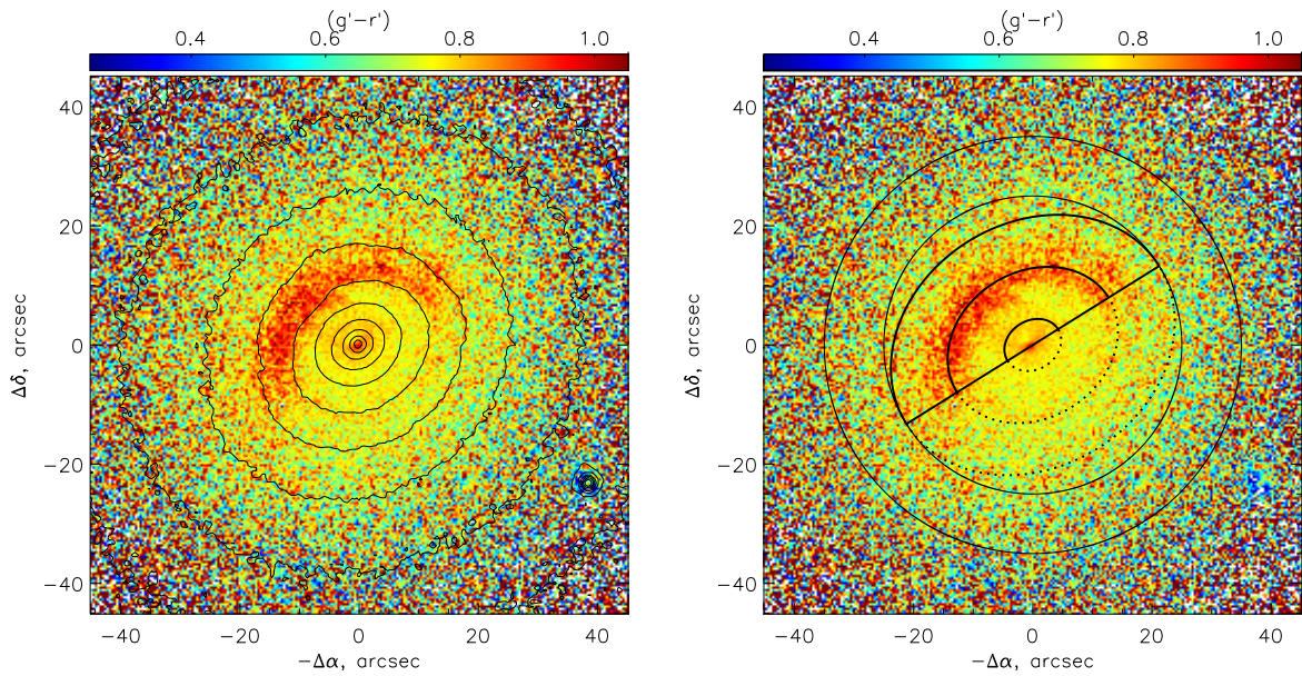
Рис. 2.5 Карта показателя цвета (g-r) для NGC 5631 по данным SDSS, на которую наложены изофоты r -изображения (слева) и схематически показана ориентация газового и звездного дисков (справа). Принятые параметры для газопылевого диска: i = 35^\circ , PA = 122^\circ .
