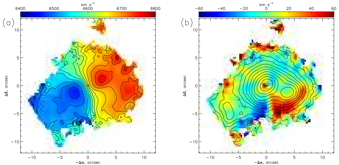
Рис. 3.12 Mrk 334. Кинематика ионизованного газа по данным ИФП в линии \text{H}\alpha . (a) – поле лучевых скоростей, (b) – остаточные скорости (наблюдения минус модель) с изофотами в линии \text{H}\alpha .
