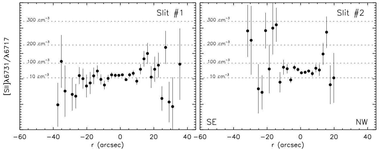
Рис. 6.10 Измерения электронной плотности по отношению линий дублета [SII] в обоих спектральных разрезах.
