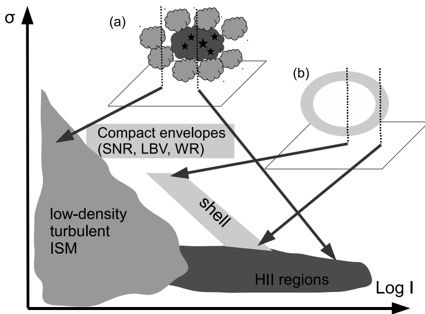
Рис. 7.8 Схема, поясняющая расположение точек на диаграмме I - \sigma . На врезках показано, как на картинную плоскость проецируется распределение яркости и дисперсия скоростей от областей HII, окруженных газом низкой плотности со значительными турбулентными движениями (a) и от расширяющейся оболочки — (b). Пунктиром показаны лучи зрения, проецирующие на картинную плоскость разные пространственные области.
