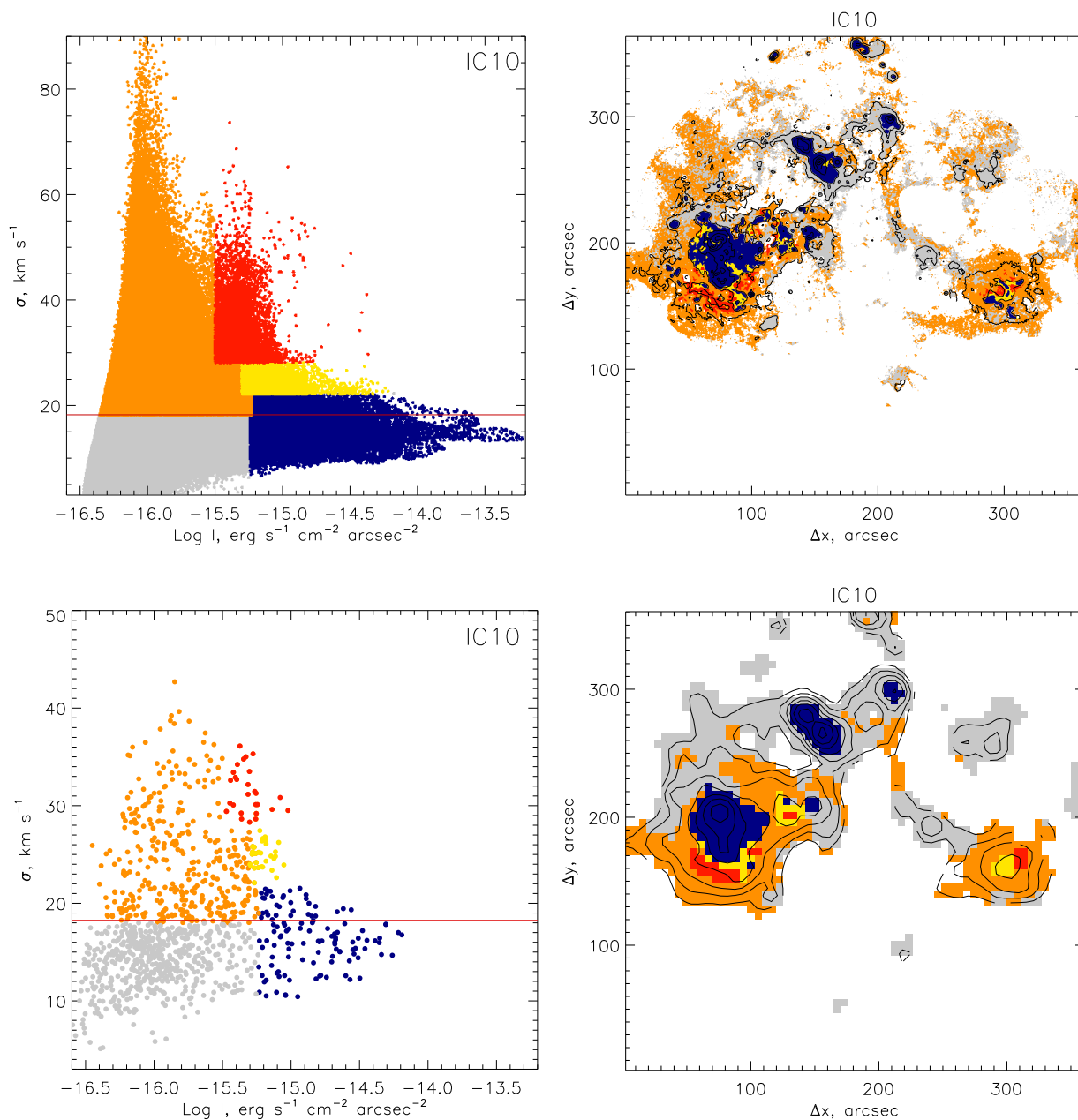
Рис. 7.6 IC10: исходные данные (вверху) и сглаженные (внизу). Слева показаны диаграммы I - \sigma . Красная горизонтальная линия отмечает величину средневзвешенной по яркости дисперсии скоростей \sigma_m . Справа показана локализация областей, выделенных разным цветом на диаграмме I - \sigma . Контуры соответствуют изофотам в линии \text{H}\alpha .
