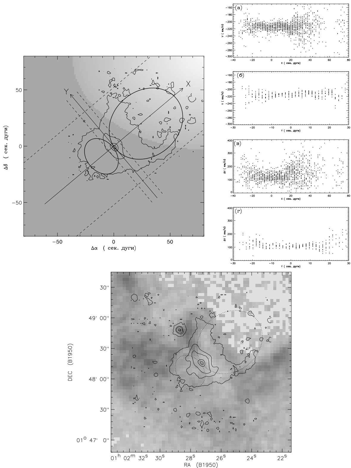
Рис. 6.1 Вверху слева — общая схема туманности S3, связанной со звездой WO. Биполя́рная оболочка обозначена двумя эллипсами. Штриховые линии показывают границы разрезов вдоль осей X и Y. Показаны изофоты в линии H \alpha , согласно наблюдениям на БТА с ИФП. Градациями серого отмечено распределение поверхностной плотности H \alpha по данным низкого разрешения (Lake & Skillman, 1989). Справа — результаты измерений скоростей (а, б) и FWHM (в, г) в линии H \alpha вдоль осей X и Y. Внизу — туманность S3 и распределение H \alpha по новым данным (Лозинская и др., 2001).
