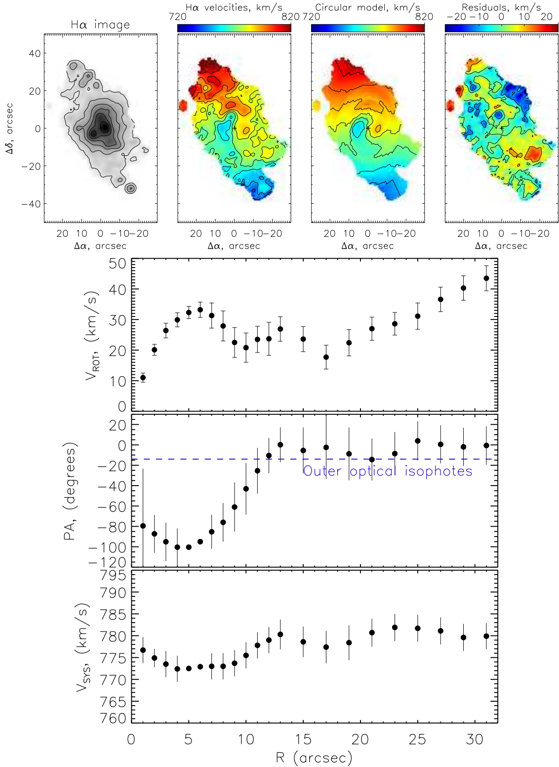
Рис. 5.7 Mrk 370. Верхний ряд – результаты наблюдения с ИФП в линии H \alpha , слева направо: изображение в эмиссионной линии, поле лучевых скоростей, модель кругового вращения, остатки после вычитания модели. Внизу – радиальные изменения параметров модели вращения.
