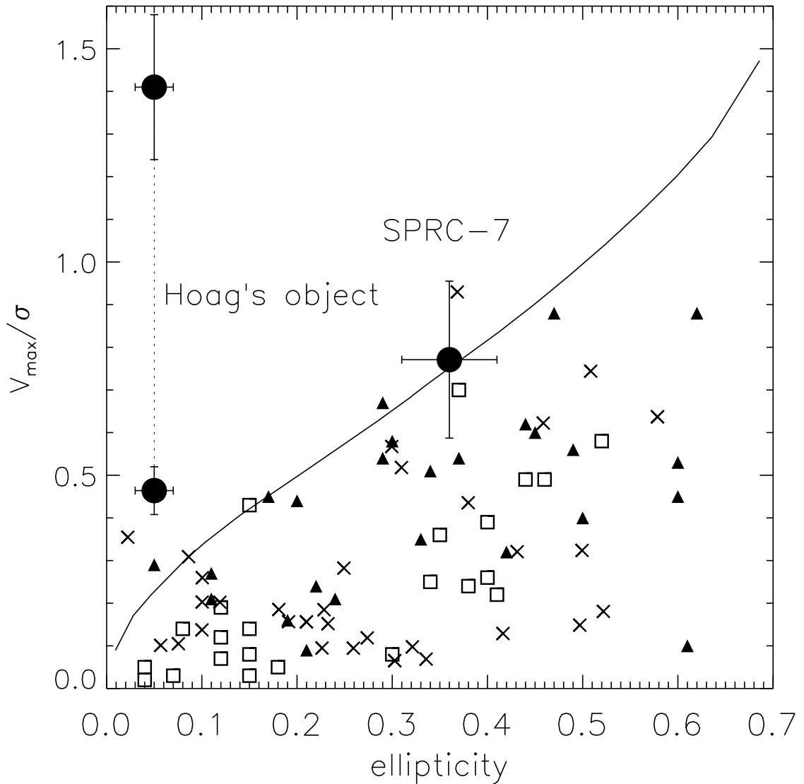
Рис. 4.8 Диагностическая диаграмма Бинни v/\sigma, \epsilon . Крестики – эллиптические галактики из Kormendy (1993), треугольниками и квадратами отмечены S0 и E галактики из выборки SAURON (Cappellari et al., 2007). Жирными кружками с усами ошибок показаны результаты наших наблюдений галактик, рассмотренных в данной главе. Для Объекта Хога приведены два значения, соединенные пунктиром – до и после исправления за наклон. Сплошная линия – теоретическая кривая для сплюснутого сфероида, поддерживаемого вращением (Kormendy, 1993)
