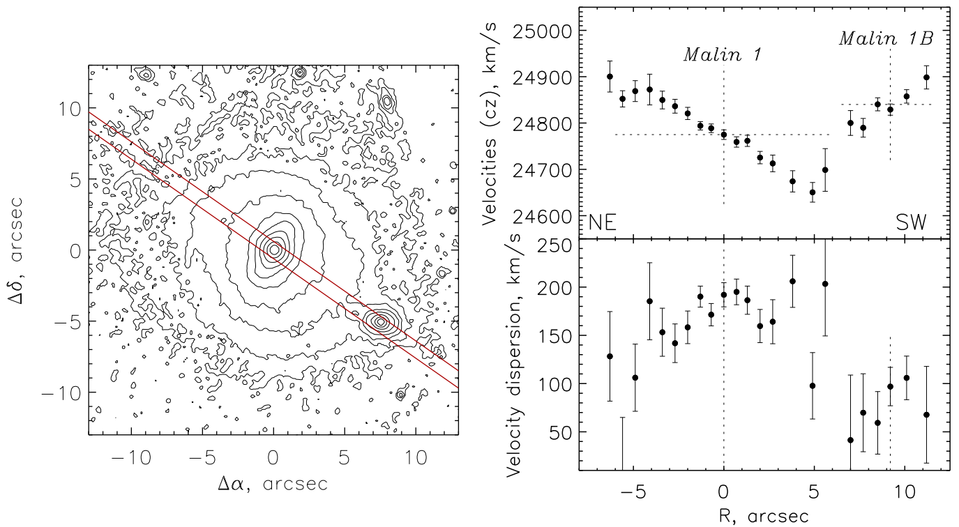
Рис. 3.5 Слева – изофоты центральной части галактики Malin 1 в полосе I , по данным WFPC2/HST. Показано положение щели спектрографа SCORPIO при наблюдений на 6-м телескопе. Справа – распределение лучевой скорости и дисперсии скоростей звезд вдоль PA = 55^\circ . Отмечены центры Malin 1 и Malin 1B.
