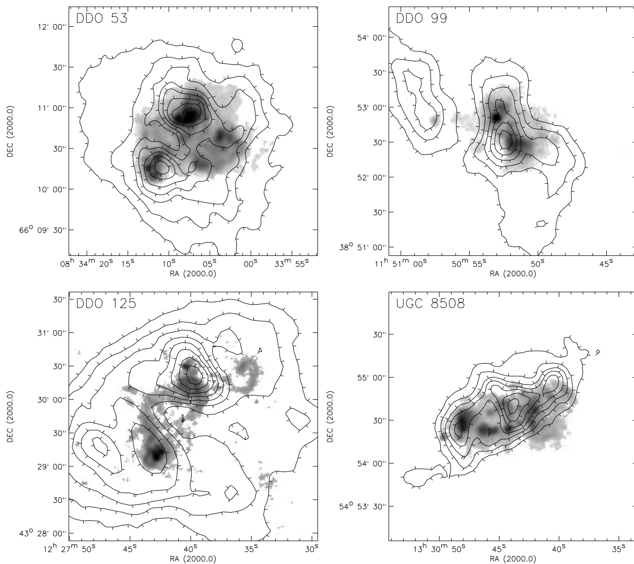
Рис. 7.9 Сравнение распределений яркости в H\alpha (серые градации) и плотности HI (контур). Данные по нейтральному водороду для DDO 53 приведены из обзора THING (Oh et al., 2011), для остальных галактик — из обзора FIGGS (Begum et al., 2008).
