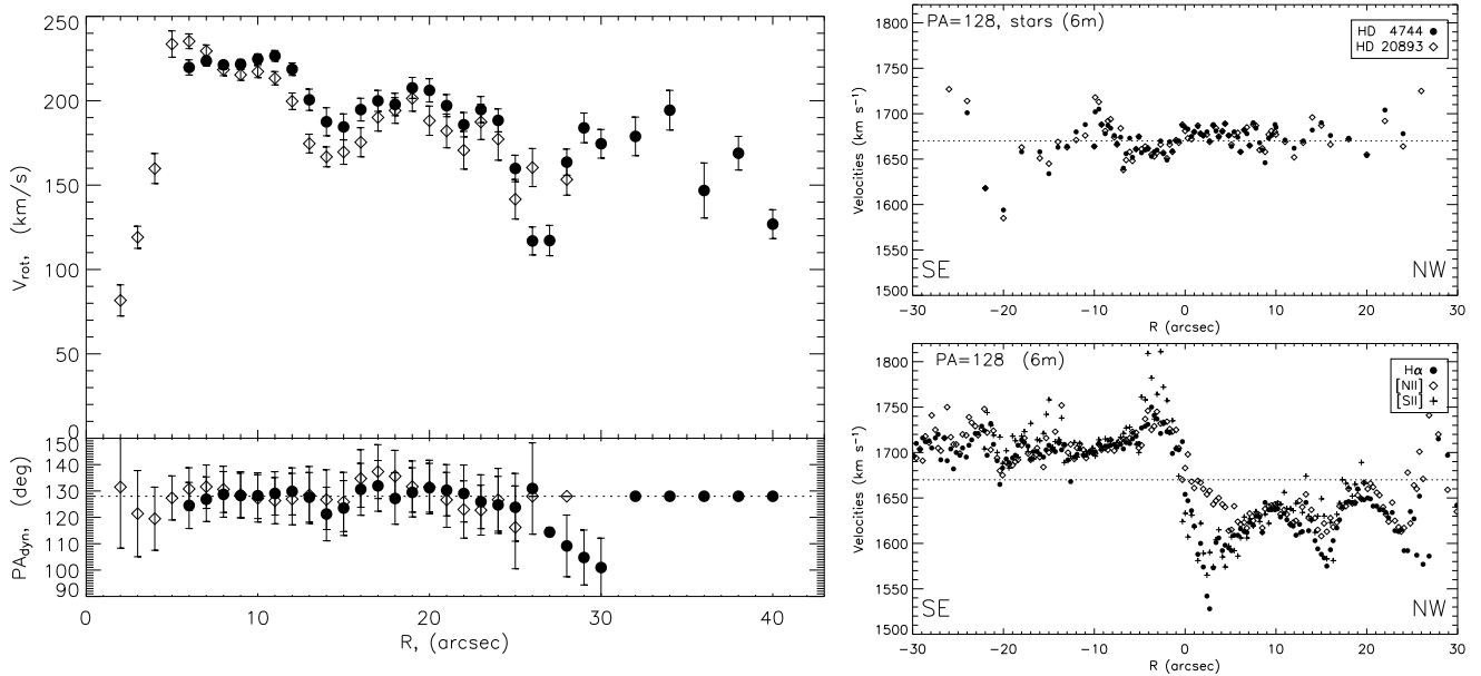
Рис. 2.7 Слева: радиальные изменения скорости вращения и PA_{kin} , измеренные по полям скоростей H\alpha (черные точки) и [NII] (ромбики). Справа: распределения лучевых скоростей вдоль щели спектрографа. Верхняя панель – звездное население (указаны два варианта используемых кросс-корреляционных шаблонов), внизу – эмиссионные линии ионизованного газа. Пунктиром показана системная скорость.
