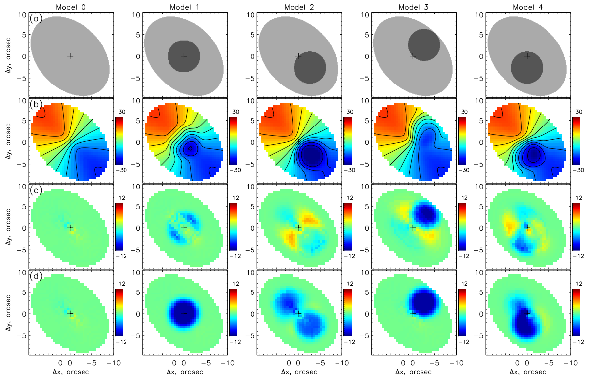
Рис. 1.9 Расширяющаяся оболочка в галактическом диске. (а) – относительные положения диска (серый цвет) и оболочки (чёрный). (b) – модельные поля скоростей, после вычитания V_{sys} = 1000 км/с. (с) – остаточные поля скоростей в Методе I, в котором разрешаются радиальные вариации PA и V_{sys} . (d) – остаточные поля скоростей в Методе II, где PA, V_{sys} = \text{const}
