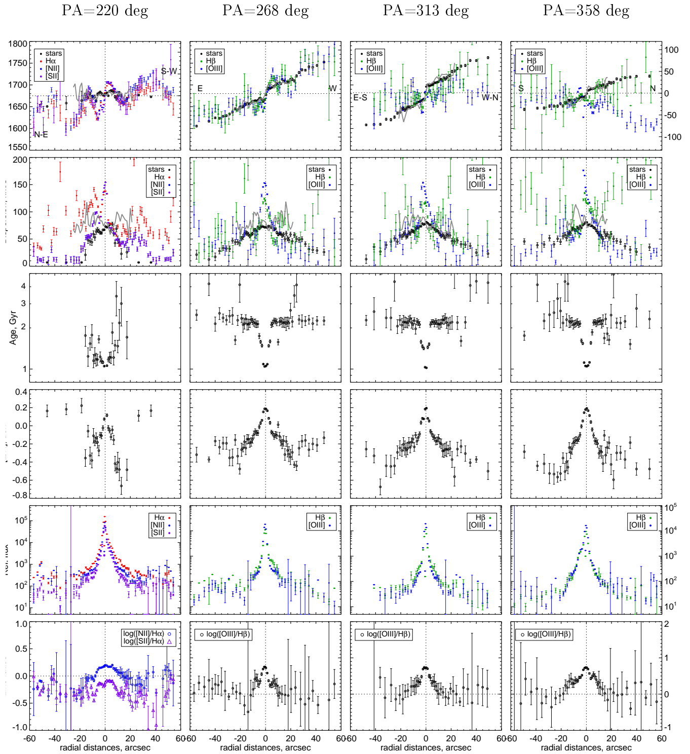
Рис. 2.9 Результаты длиннощелевых наблюдений. Каждый столбец соответствует позиционному углу, указанном сверху, для PA = 220^\circ данные приведены для “красного” диапазона, в остальных случаях - для “зеленого”, в котором кинематика звезд измеряется лучше. Сверху вниз: радиальные профили лучевых скоростей, дисперсии скоростей, возраста, металличности звезд, интенсивностей эмиссионных линий (в условных единицах) и отношения потоков в линиях.
