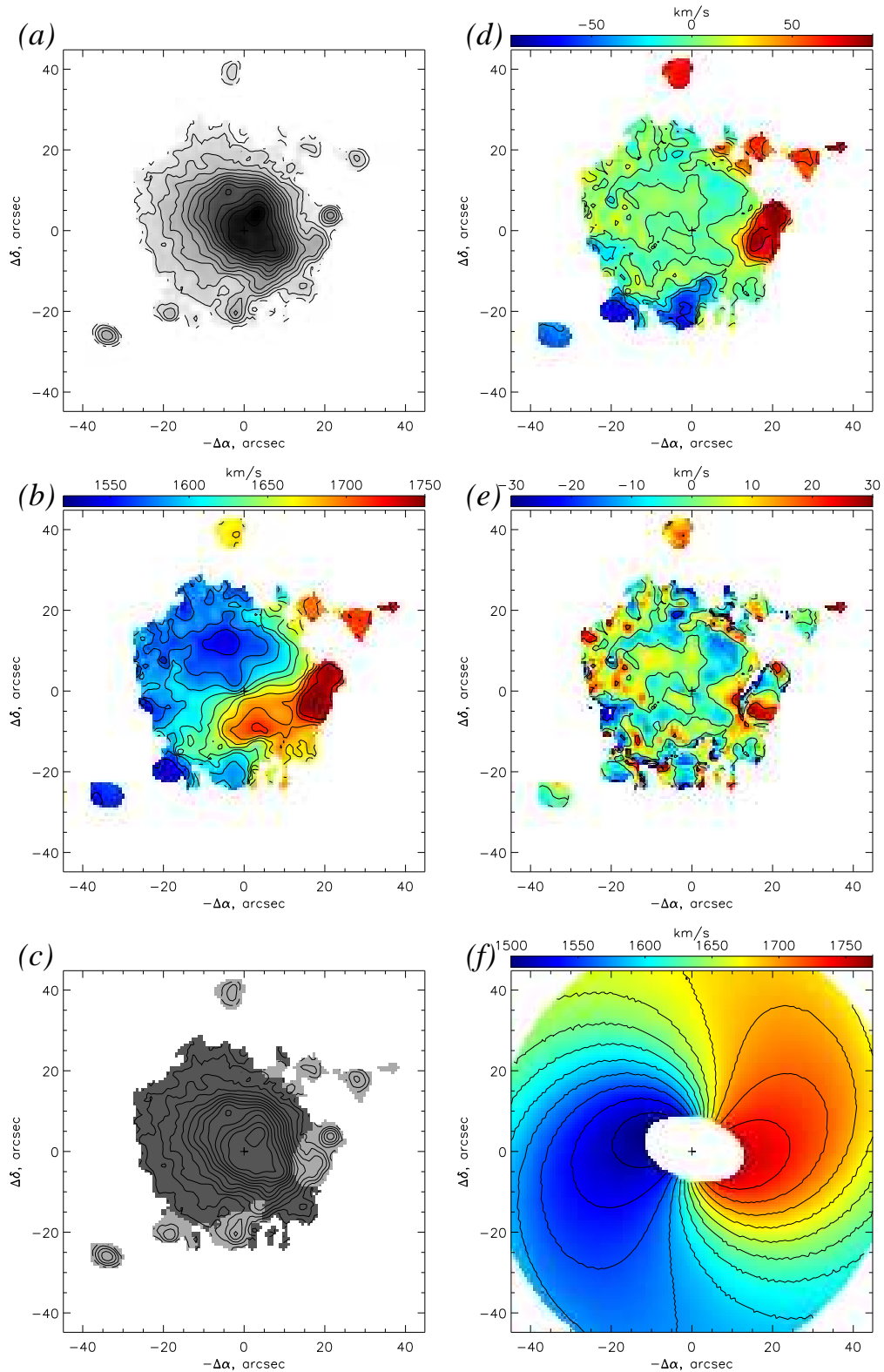
Рис. 4.1 M33: распределение интенсивности в линии H \alpha в логарифмической шкале (a), поле лучевых скоростей (b), схема разделения галактики (c) на внутренний диск (темное) и внешние филаменты (светлое), с наложенными изофотами в линии H \alpha . Карты остаточных лучевых скоростей: для круговой модели вращения внутреннего диска (d), для раздельного учета вращения внутренних и внешних областей (e). Поле скоростей филаментов в двумерной модели изогнутого диска (f).
