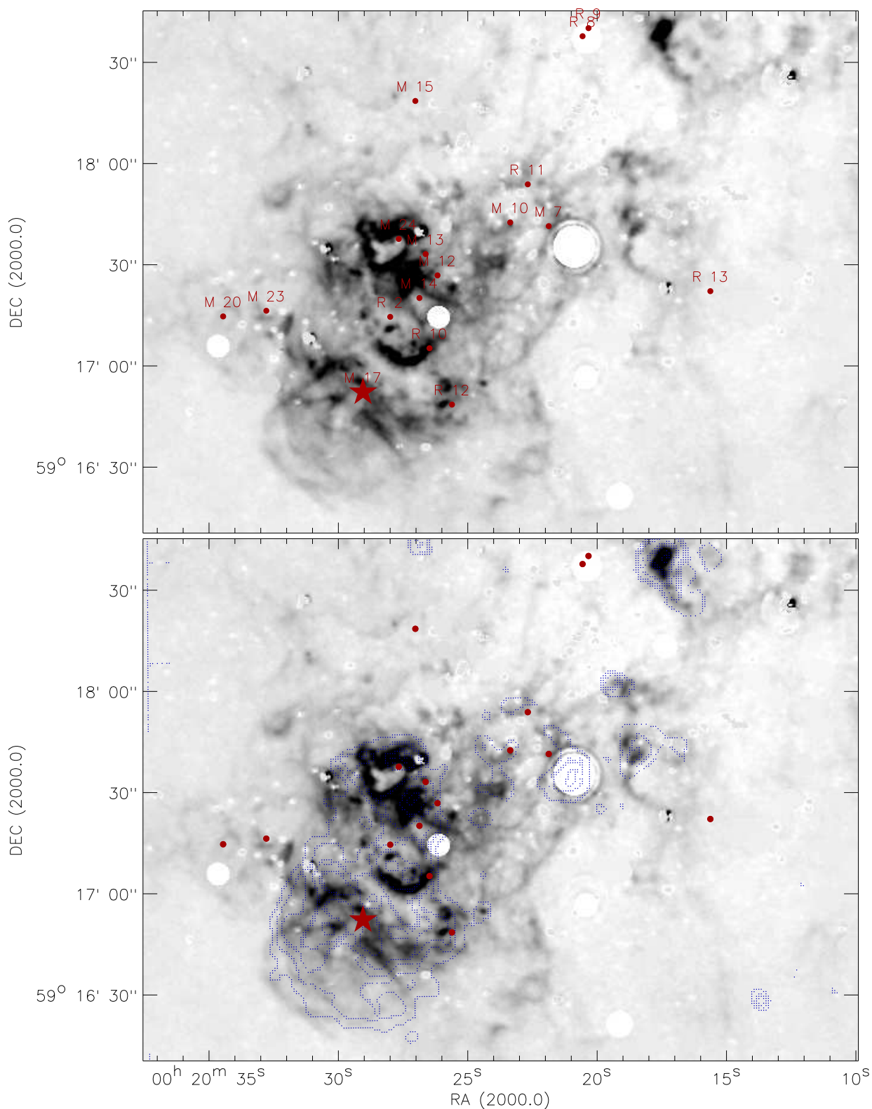
Рис. 6.4 Вверху: изображение комплекса звездообразования в IC 10 в эмиссионном дублете [\text{SII}]\lambda 6717, 6731 , полученное на 6-м телескопе со SCORPIO. Красными кружками отмечены спектрально-подтвержденные звезды WR из списков Royer et al. (2001) и Massey & Holmes (2002). Компактный рентгеновский источник X-1 (черная дыра в паре со звездой WR M17) показан звездочкой. Внизу: то же самое, совмещенное с радиоизофотами на 20 см (Yang & Skillman, 1993), отмечающих синхротронную сверхоболочку.
