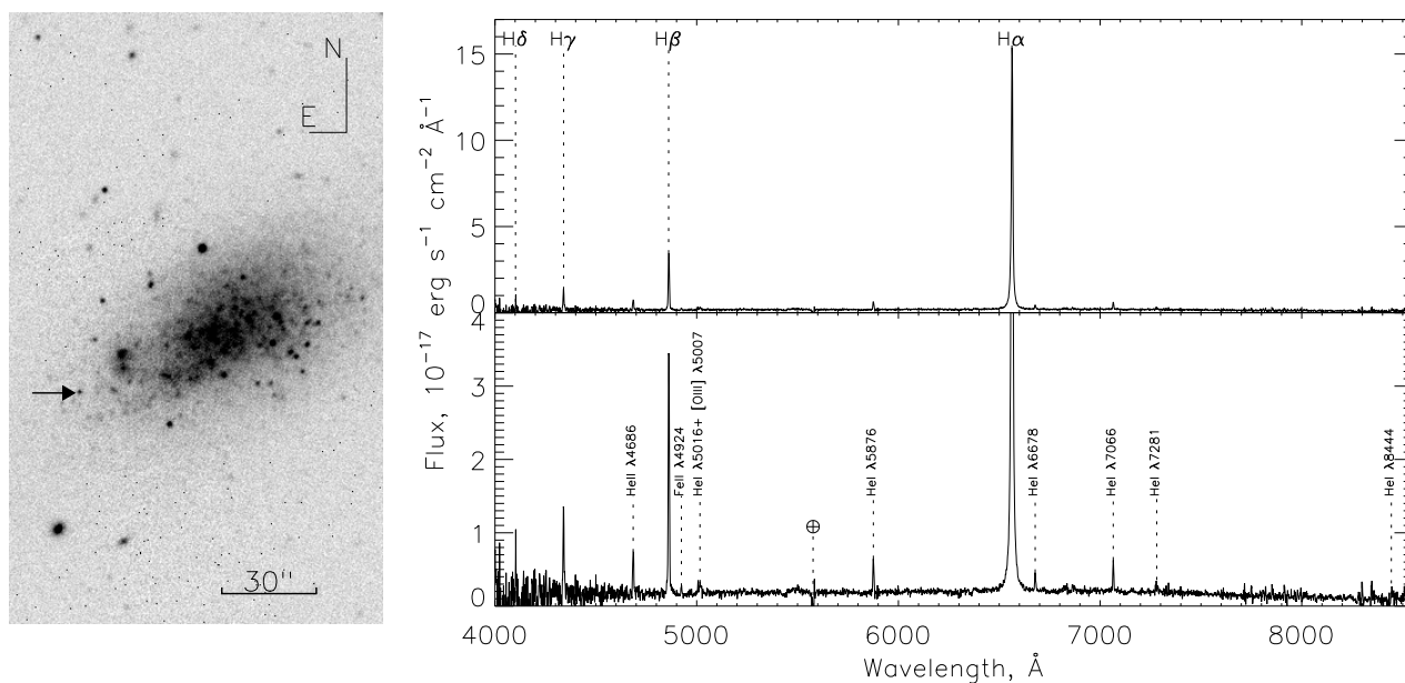
Рис. 7.4 Кандидат в LBV в UGC 8508. Слева – изображение в фильтре r из SDSS DR8, звезда отмечена стрелочкой. Справа – спектр звезды в двух вариантах шкалы интенсивностей, показаны основные эмиссионные линии.
