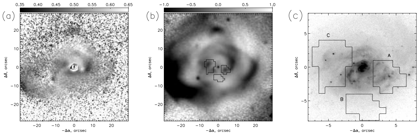
Рис. 3.8 Распределение показателя цвета (V-R) во внутренних областях галактики (а), остаточные яркости для этой же области (b) и изображение из архива HST (с), полученное камерой PC в фильтре F606W. На рисунках (b) и (с) контурами показаны границы конденсаций, выделенных по наблюдениям с MPFS.
