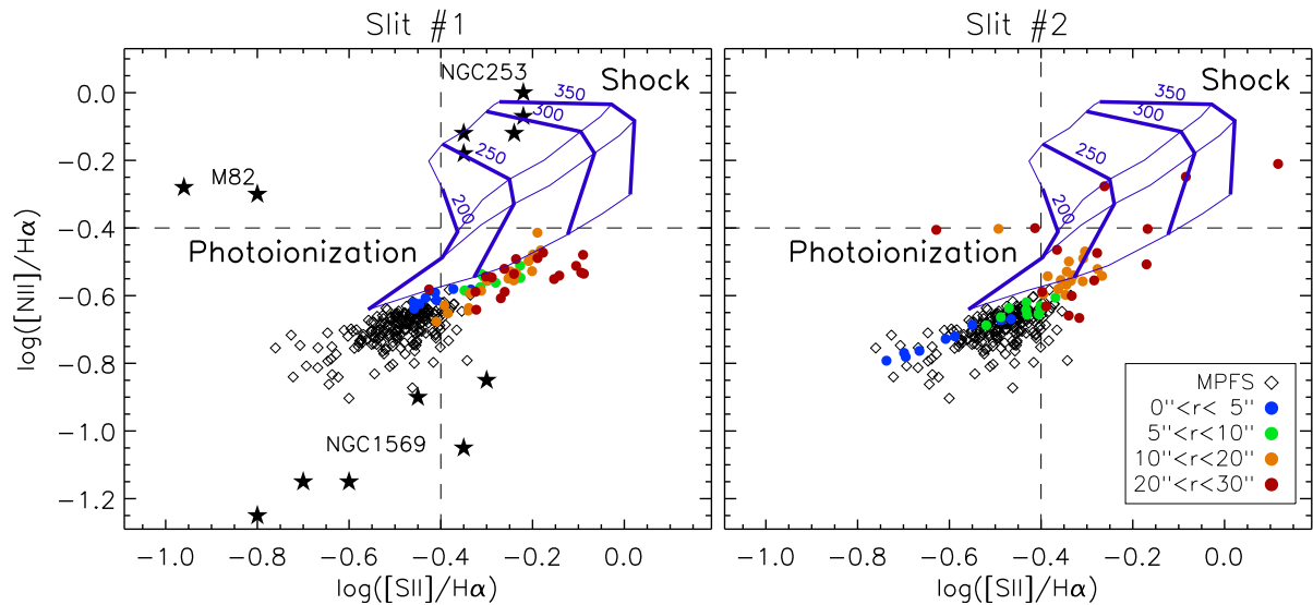
Рис. 6.9 Диаграмма отношения потоков [\text{NII}]/\text{H}\alpha – [\text{SII}]/\text{H}\alpha . Пунктир разделяет области с различными механизмами ионизации. Нанесена сетка ионизационных ударных моделей (Allen et al., 2008), где тонкие линии соответствуют значениям магнитного параметра 0, 1, 2, 4 \mu\text{G cm}^{2/3} (снизу вверх), а толстые линии – подписанным скоростям ударной волны (в км/с). Кружками показаны измерения вдоль разрезов 1 (слева) и 2 (справа). Цвета соответствуют разным расстояниям от плоскости галактики. Ромбами показаны результаты MPFS для околоядерной области. Звездочками на левом рисунке отмечены измерения для областей галактического ветра в M82, NGC253 и NGC1569.
