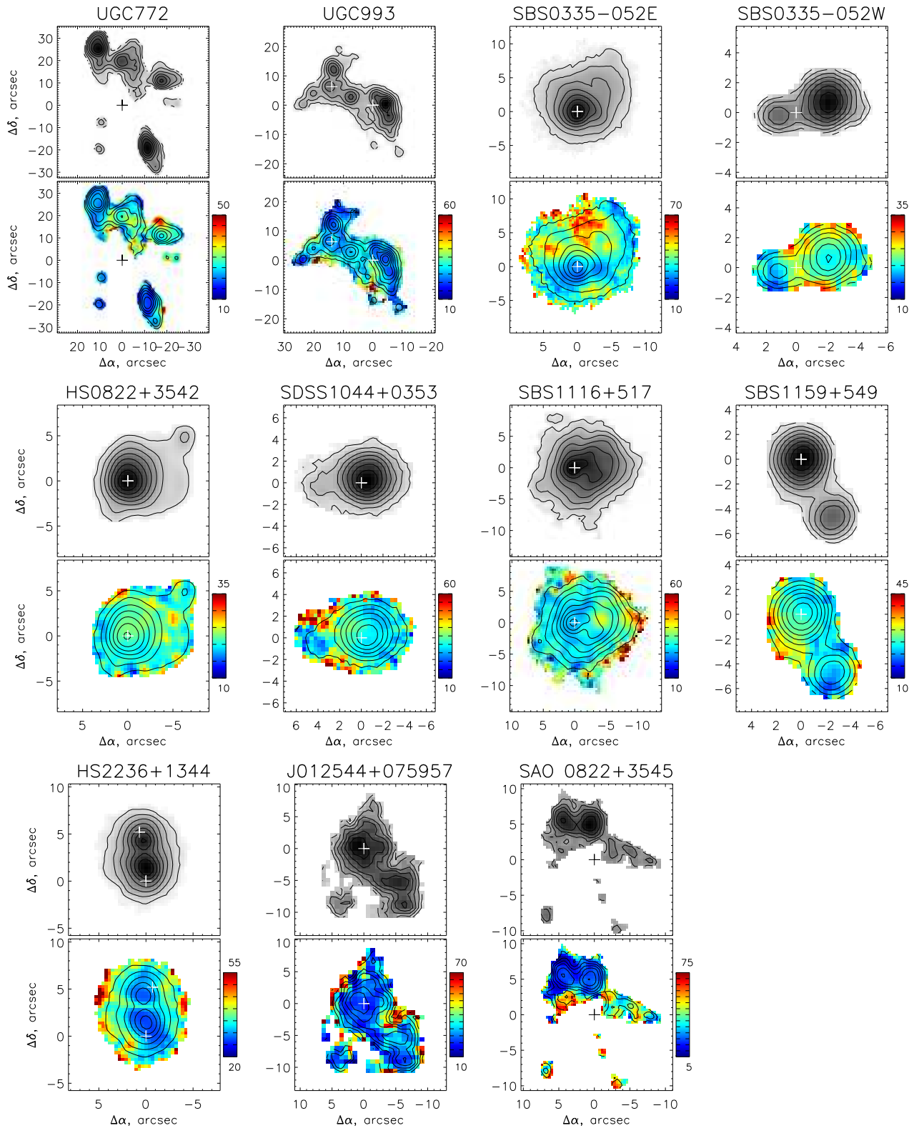
Рис. 7.1 Карты распределения интенсивности в линии H\alpha (серые градации) и дисперсии скоростей (цветные) для выборки карликовых галактик с пониженной металличностью (Moiseev et al., 2010b). Крестиком помечен центр вращения, определенный из поля скоростей (по два для взаимодействующих объектов), шкала – в км/с. Контурами показаны уровни интенсивности H\alpha в логарифмической шкале.
