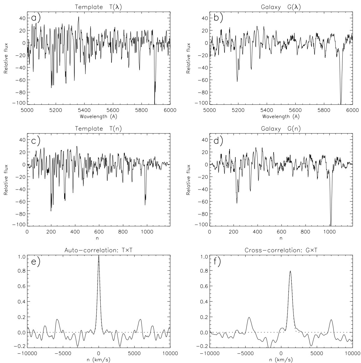
Рис. 1.7 Кросс-корреляционный метод (Moiseev, 2001a). a,b – спектры звезды класса KIII и галактики NGC 2950, континуум вычтен; c, d – спектры в логарифмической шкале с шагом 50 км/с; e,f – автокорреляционная и кросс-корреляционная функции, пунктиром показана аппроксимация пиков гауссианой.
