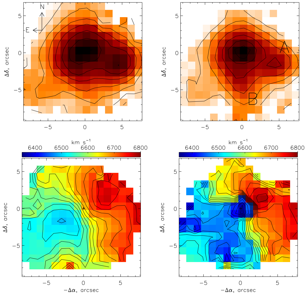
Рис. 3.6 Mrk 334. Изображения (вверху) и поля скоростей (внизу) в эмиссионных линиях по данным наблюдений с MPFS в линии \text{H}\alpha (слева) и [\text{OIII}]\lambda\lambda 4959, 5007 (справа). Отмечены области “А” и “В”.
