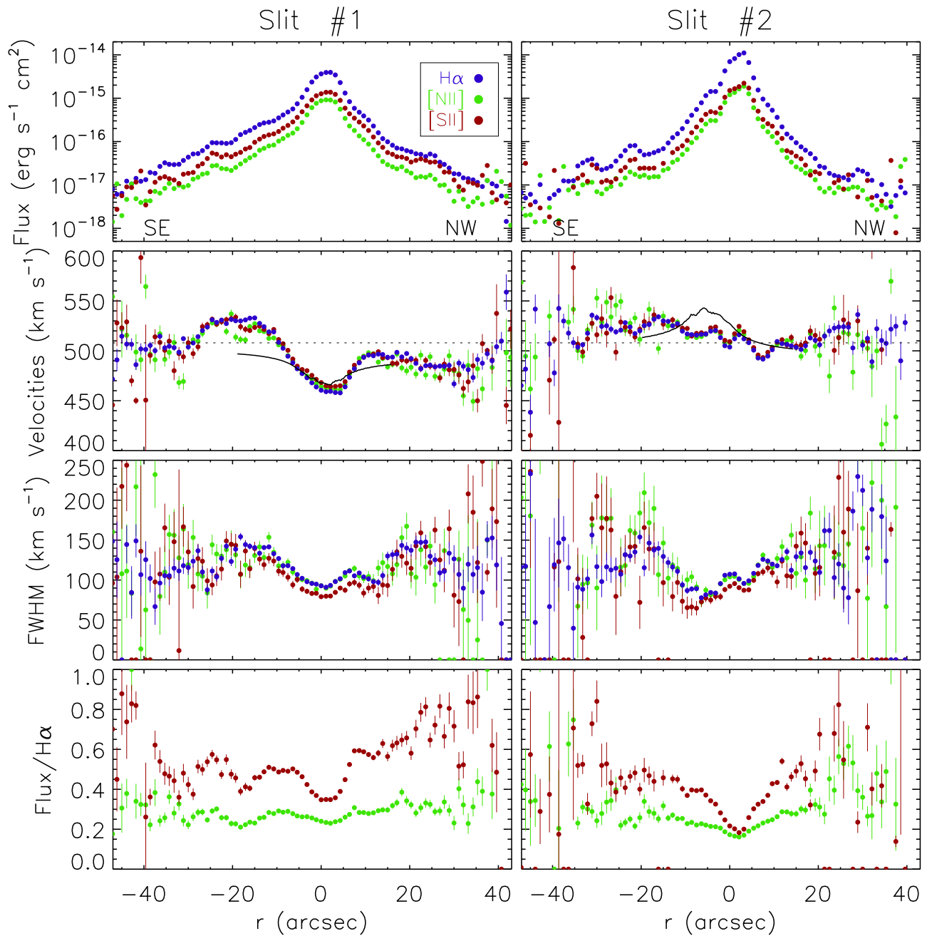
Рис. 6.8 Изменение вдоль щели параметров эмиссионных линий H\alpha , [NII]\lambda 6583 и [SII]\lambda 6717+6731 в NGC 4460. Слева – разрез 1, справа - разрез 2. Сверху вниз: поверхностная яркость, лучевая скорость, полуширина (скорректированная за ширину инструментального профиля) и отношение потока в линиях относительно H\alpha . На графиках для скоростей пунктиром помечена системная скорость (по данным MPFS), а сплошной линией – разрез через модельное поле скоростей.
