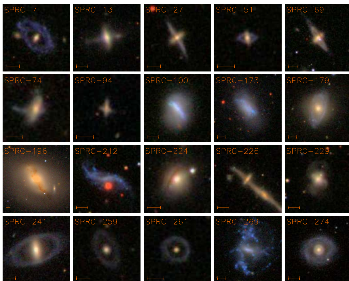
Рис. 4.15 Характерные изображения кандидатов в ГПК – комбинация изображений в фильтрах g, r, i по данным SDSS DR8. Представлены разные типы объектов (сверху вниз – лучшие кандидаты, хорошие, родственные объекты и кольца видимые плашмя). Мерная линейка соответствует угловому размеру 10'' .
