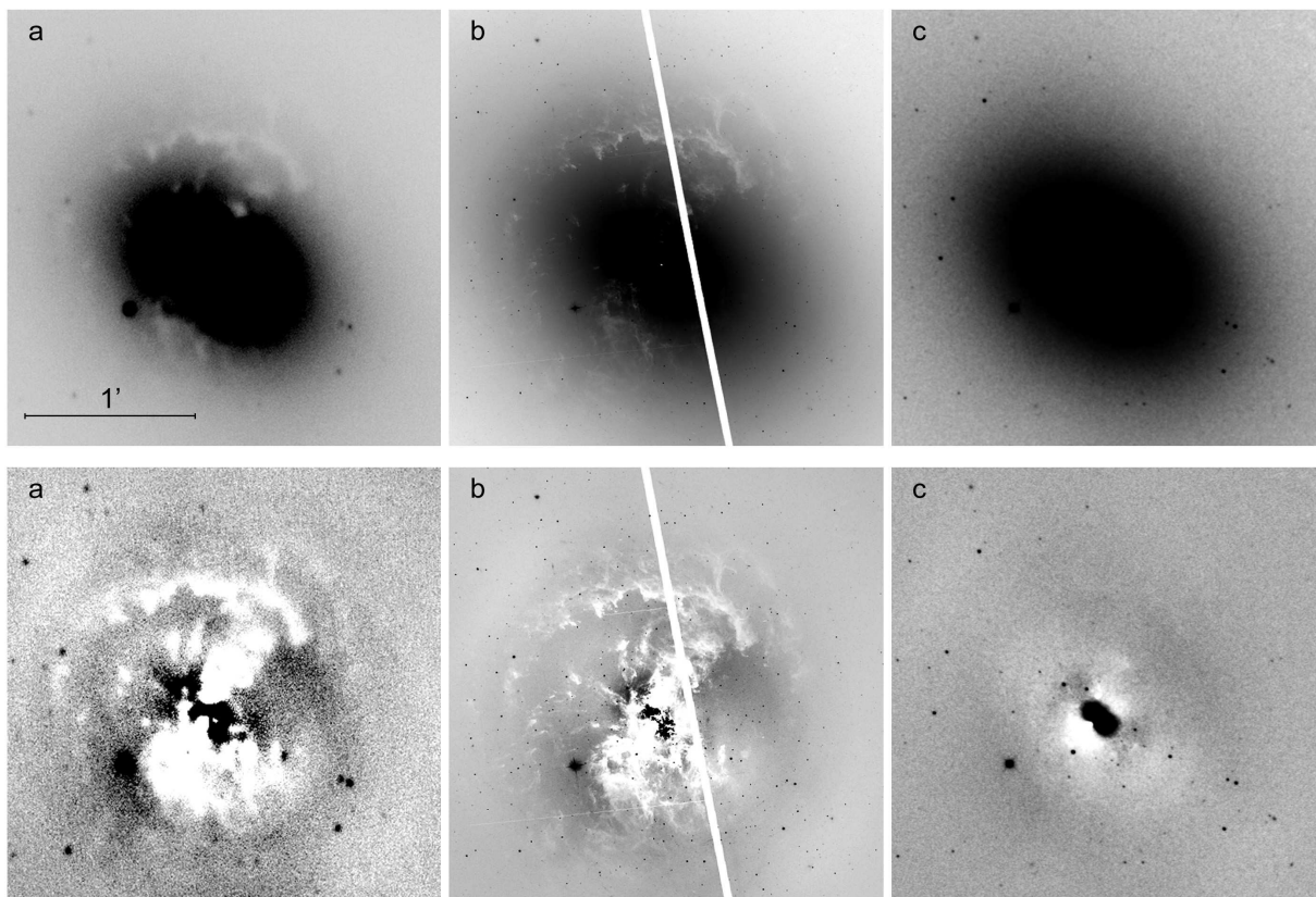
Рис. 2.2 Изображения NGC 1316. Верхний ряд (a) фильтр B (СТЮ, 0.9m), (b) фильтр V (F555W) HST/ASC, (c) фильтр Ks (SOFI/NTT). Нижний ряд : Остатки после вычитания 2D-модели распределения яркости в тех же фильтрах. Более темные градации соответствуют положительным избыткам.
