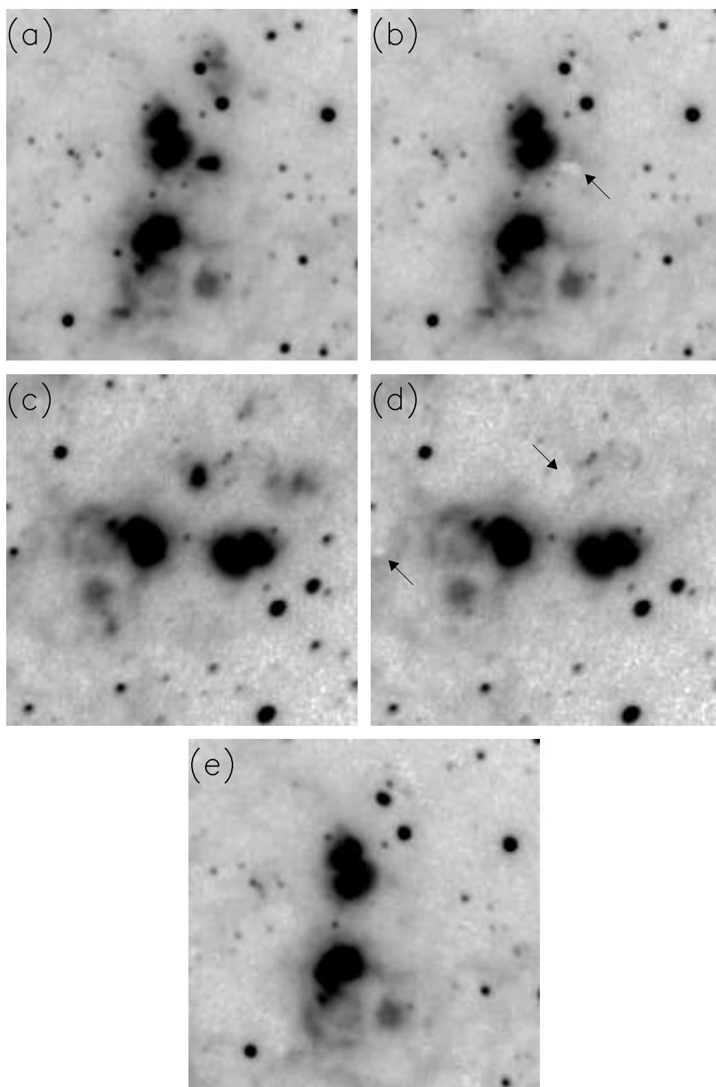
Рис. 1.4 Сумма каналов в кубах данных для галактики IC 10 в линии H\alpha : (a) исходное изображение в первом кубе; (b) после вычитания бликов, стрелка указывает на области с неудовлетворительным качеством вычитания; (c) изображение в кубе, полученном после поворота поля зрения на 90^\circ ; (d) вычитание бликов из второго куба; (e) сумма обоих наборов данных.
