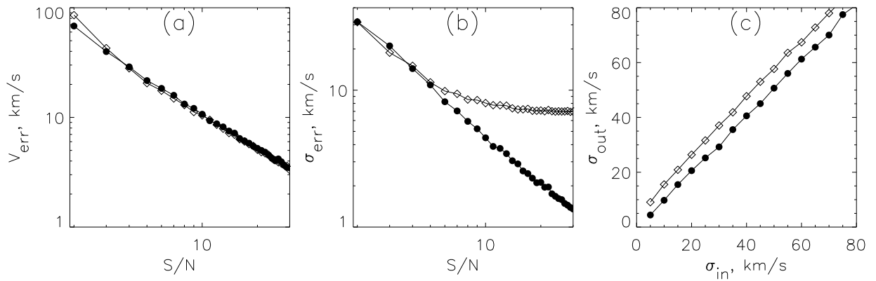
Рис. 1.6 Моделирование ошибок измерения кинематических параметров (по уровню 1\sigma ). Расчет проводился для IFR501. Ромбики – аппроксимация гауссианой, черные кружки – профилем Фойгта. (а) зависимость ошибки измерения лучевой скорости от уровня отношения сигнал-шум, средняя величина дисперсии скоростей составляла 50 км/с; (б) зависимость ошибки измерения дисперсии скоростей от уровня отношения сигнал-шум при тех же условиях; (с) сравнение исходной и измеренной дисперсии скоростей (для S/N = 20 )
