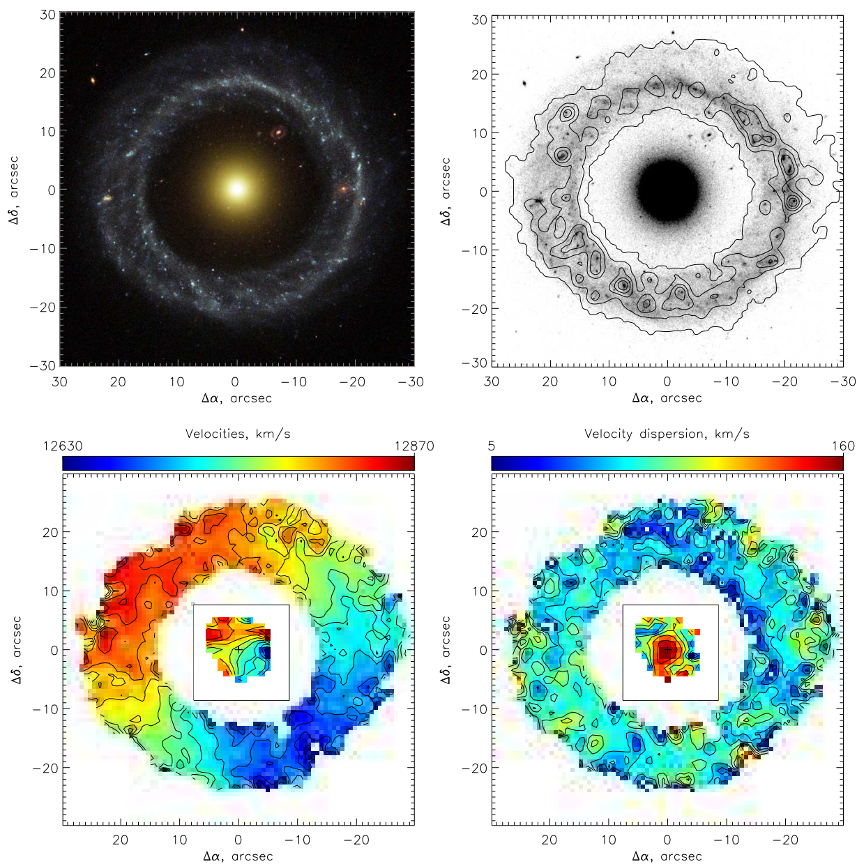
Рис. 4.9 Объект Хога. Верхний ряд – цветное изображение из Hubble Heritage (телескоп HST, камера WFPC2) и изофоты в линии H\alpha (ИФП) нарисованные поверх изображения HST в фильтре F606W. Нижний ряд – кинематика звезд в центре (MPFS) и ионизованного газа в кольце (ИФП). Слева – поле лучевых скоростей, справа – дисперсия скоростей. Квадратом показано поле зрения спектрографа MPFS.
