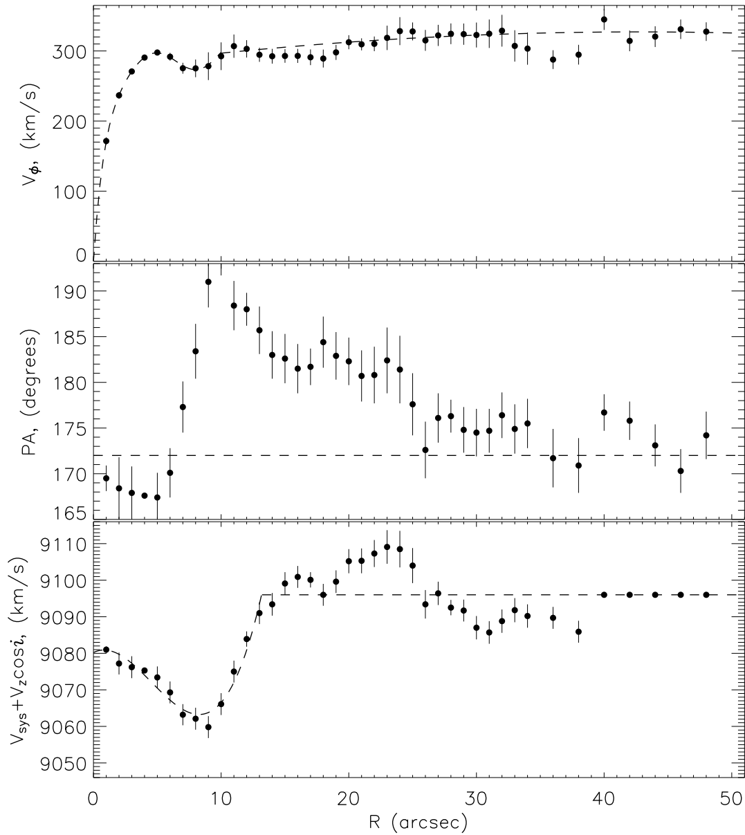
Рис. 3.2 Анализ поля скоростей Agn 10 в рамках модели квазикругового вращения. Сверху вниз: скорость вращения, позиционный угол, системная скорость. Пунктиром показана аппроксимация радиального изменения параметров, принятая для построения модельного поля скоростей, показанного на предыдущем рисунке.
